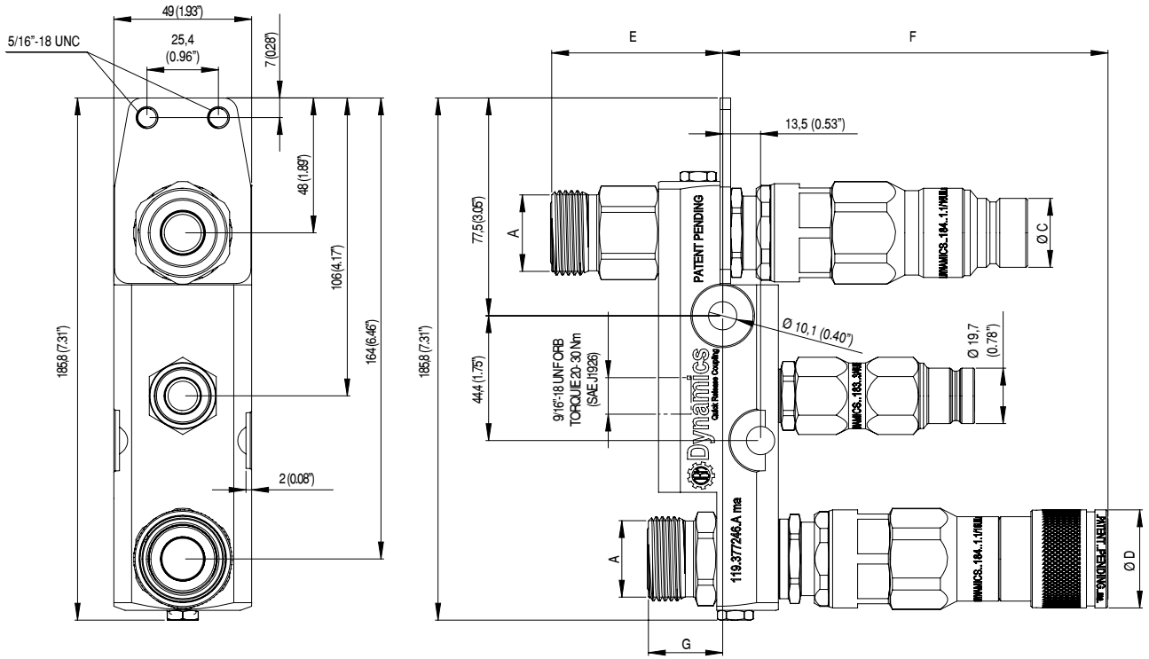
Bloco com Engates com Válvula de Despressurização / Bloque de Acoplamiento con Válvula de Despressurización / Decompression Block Coupler
