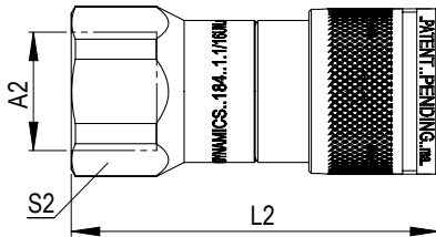
Engate Rápido Fêmea tamanho 12,7 (1/2") ou 19,1 (3/4") Acople Rápido Hembra tamanho 12,7 (1/2") o 19,1 (3/4") Female Quick Coupler size 12,7 (1/2") or 19,1 (3/4")
